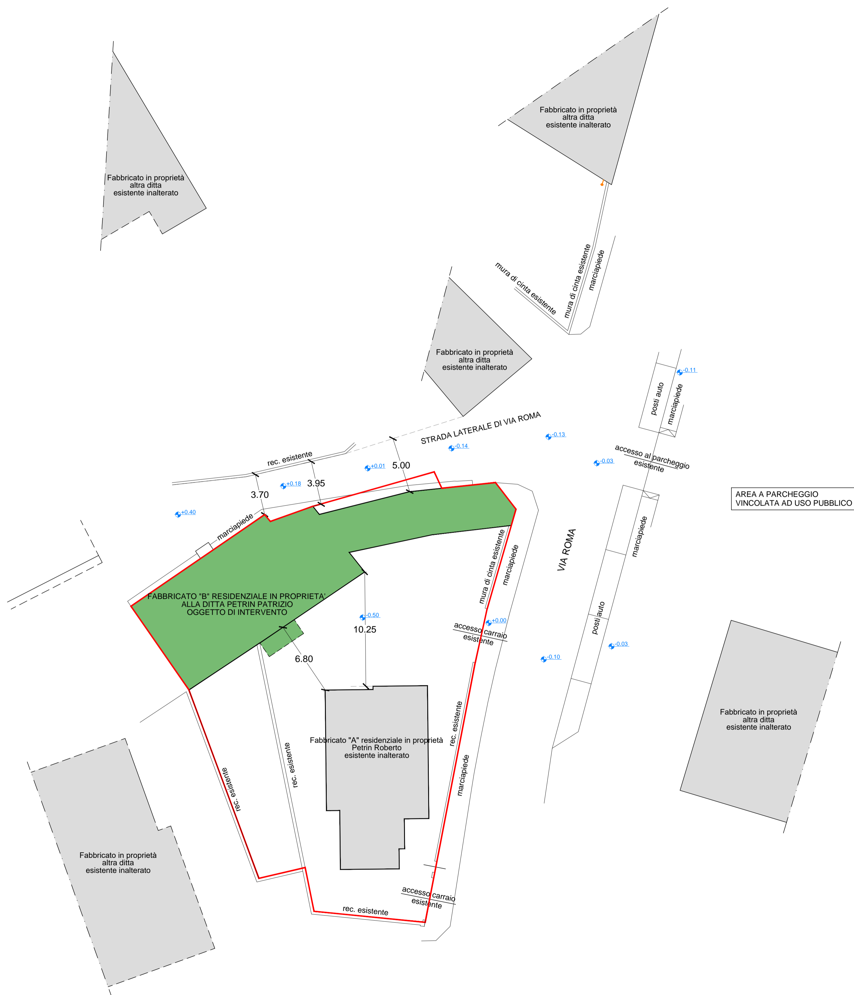
PLANIMETRIA GENERALE DELLO STATO DI FATTO IN SCALA 1:200
